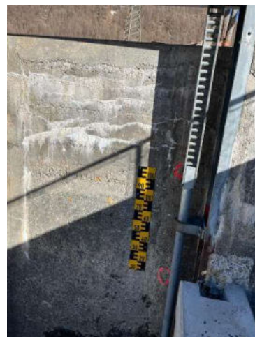
Beim Ausgleichsbecken in der Egga wurde der Überlauf saniert und der Grundablassschieber erneuert.
